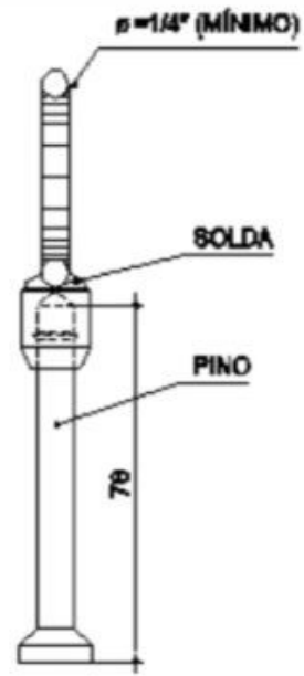
2 TRANSPASSADOR DE CABO - CORTE AA 2 CBR: MEDIDAS EM MILÍMETROS
